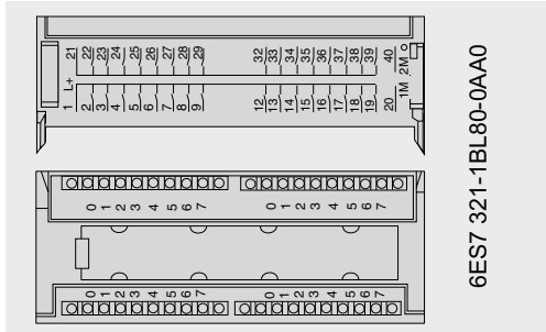
Bild 2/1 Digitaleingabebau- gruppe SM 321-1BL80
